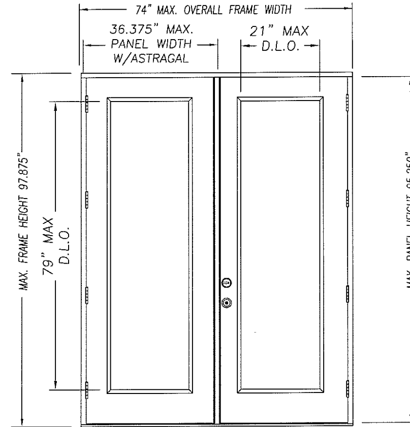
DOUBLE DOOR UNIT
